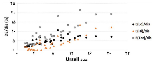
شکل ۹: تغییرات نسبت افزایش انرژی فرکانس‌های بالا، پایین و مجموع به انرژی مستهلک شده در اثر شکست در برابر عدد Ursell
