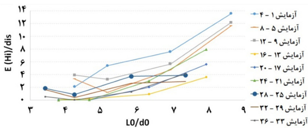
شکل ۷: تغییرات نسبت افزایش انرژی فرکانس‌های بالا به انرژی مستهلک شده در حین شکست موج در برابر متغیر \left(\frac{L_0}{dep0}\right)
