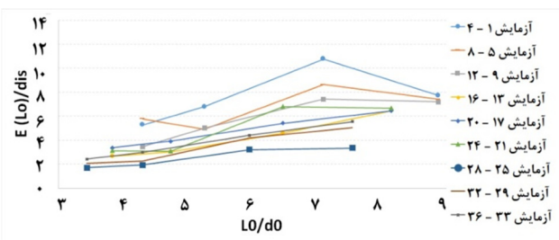
شکل ۸: تغییرات نسبت افزایش انرژی فرکانس‌های پایین به انرژی مستهلک شده در حین شکست موج در برابر متغیر \left(\frac{L_0}{dep0}\right)
