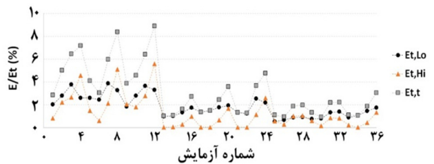
شکل ۱۰: نسبت انرژی‌های منتقل شده به فرکانس‌های بالا، پایین و مجموع آن به کل انرژی امواج در هنگام تولید
