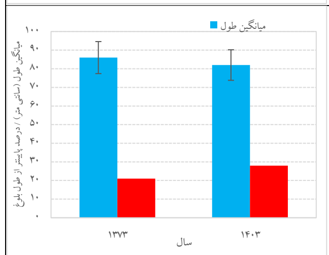
شکل ۳: درصد فراوانی طولی، میانگین طول و درصد پایین تر از بلوغ ماهی گالیت طی سال های ۱۳۷۳ و ۱۴۰۳ در آب های شمالی دریای عمان (استان سیستان و بلوچستان)
