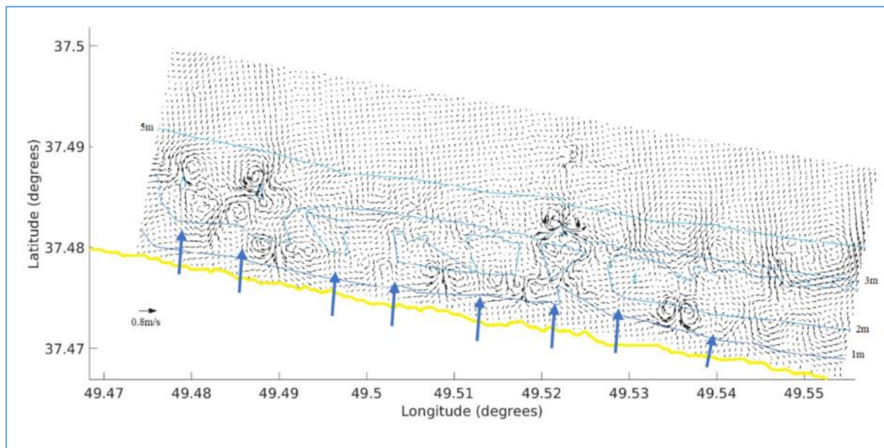
شکل ۷: جریان‌های ساحلی حاصل از مدلسازی جریان متوسط عمقی در سواحل انزلی. پیکان‌ها محل وقوع جریان شکافنده را نشان می‌دهند.
