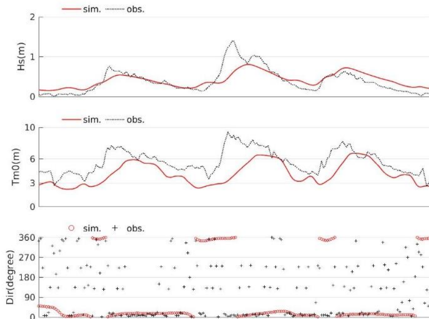
شکل ۵: مقایسه سری زمانی مشخصات امواج حاصل از مدلسازی با مقادیر اندازه‌گیری در ایستگاه B5. خط چین سیاه و + نماینده مقادیر اندازه‌گیری و خط پر قرمز و 0 نشان‌دهنده مقادیر شبیه‌سازی شده از مدل هستند Fig. 5: Comparison of the time series of modeling waveforms with the measured values at station B5, the black dashed line and + represent the measured values and the red dashed line, and 'o' represent the simulated values of the model
