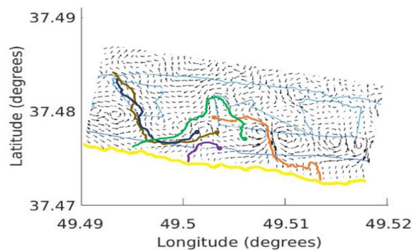
شکل ۶: مقایسه نتایج مدلسازی با ردیابی جریان‌های شکافنده با استفاده از دریغتر در سواحل انزلی Fig. 6: Comparison of modeling results by tracking rip currents using drifter in Anzali beaches
