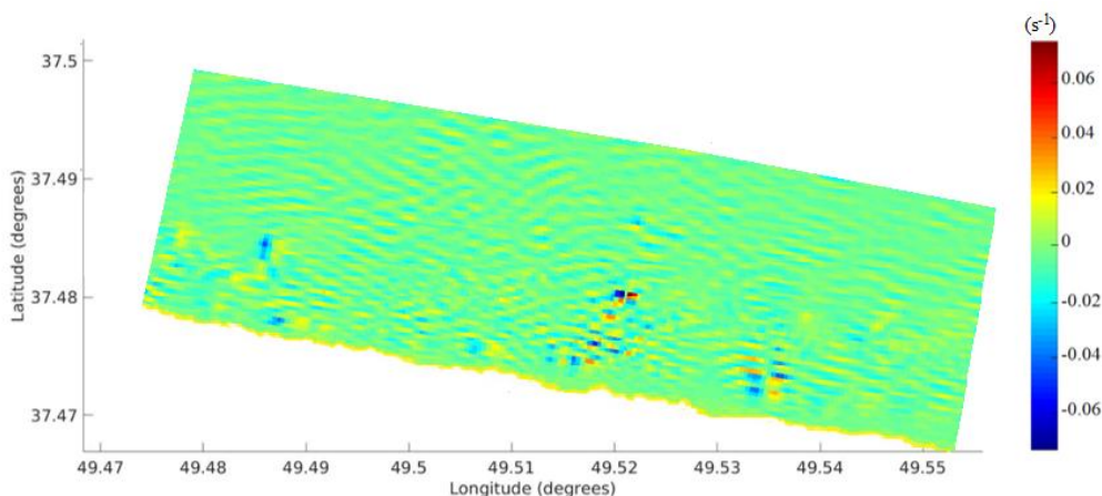
شکل ۸: میدان ورتیسیتته حاصل از مدلسازی جریان در سواحل انزلی
