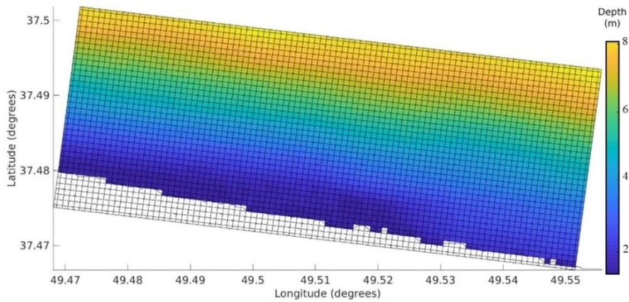
شکل ۴: شبکه محاسباتی مدل در سواحل انزلی با رزولوشن افقی ۲۰ متر. سلول‌های شبکه جهت نمایش بهتر با گام ۴:۱ ترسیم شده‌اند Fig. 4: Model computing domain in Anzali beaches with a horizontal resolution of 20 meters. The grid cells are plotted in 4: 1 for better display
