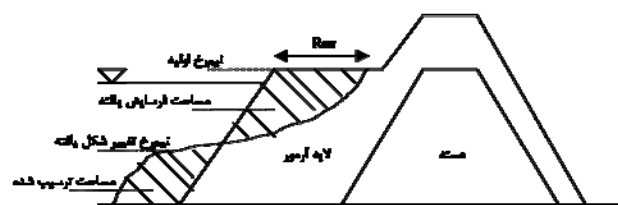
شکل ۱- موج‌شکن سکویی
