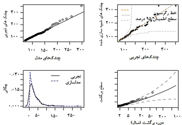
شکل ۷: برازش رویکرد تابع توزیع پارتوی تعمیم‌یافته بر اساس برآورد درست‌نمایی بیشینه در ایستگاه بندر انزلی
