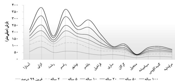
شکل ۸: نمودار آستانه بارش‌های فرین (۹۹٪) و سطح بارش‌های فرین سواحل جنوبی دریای خزر با دوره‌های برگشت ۲ تا ۱۰۰ ساله
