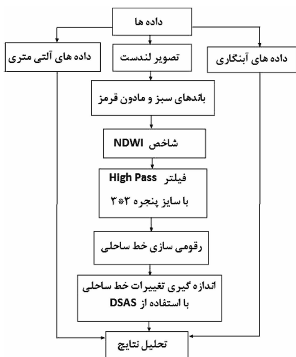
شکل ۳: چارچوب فرایند پایش تغییرات خط ساحلی
