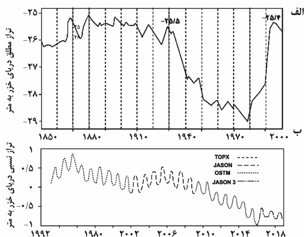
شکل ۲: الف) تراز مطلق دریای خزر بر اساس ایستگاه آب‌نگاری باکو بین سال‌های ۱۸۵۰-۲۰۰۰؛ ب) تراز نسبی دریای خزر بر اساس داده‌های ماهواره‌ای بین سال‌های ۱۹۹۲-۲۰۱۸ (عبداللهی کاکرودی، ۱۳۹۲).
