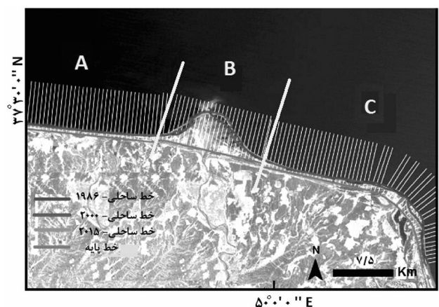
شکل ۵: ترانسکت‌های عمود بر خط مبنا و خطوط ساحلی در دلتای سفیدرود، باند ۴ تصویر TM در سال ۱۹۸۶.
