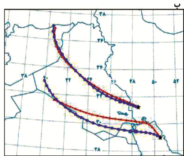
شکل ۷: برون‌دادهای الف) دید افقی مدل DREAM؛ ب) مسیر حرکت گرد و خاک مدل HYSPLIT (خط کم‌رنگ ارتفاع ۷۰۰ و خط پررنگ ارتفاع ۱۵۰۰ متری)، ۱۸ فوریه ۲۰۱۷
