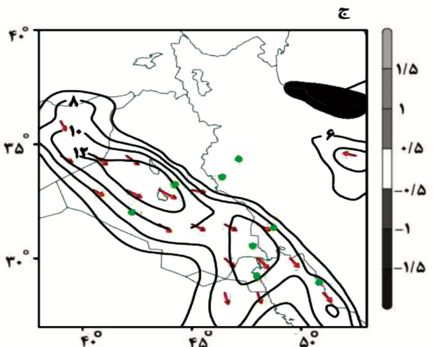
شکل ۴: گرته‌های الف) فشار میانگین تراز دریا بر حسب hPa (خطوط توپر)، ارتفاع ژئوپتانسیلی تراز ۵۰۰ hPa بر حسب متر (خطوط به صورت خط چین) و پیکان‌های باد ده متری؛ ب) تصویر ماهواره MODIS؛ ج) سرعت باد بر حسب m/s (خطوط توپر) و مولفه قائم سرعت باد بر حسب pa/s (مناطق سایه زده) برای روز ۲ سپتامبر ۲۰۱۵
