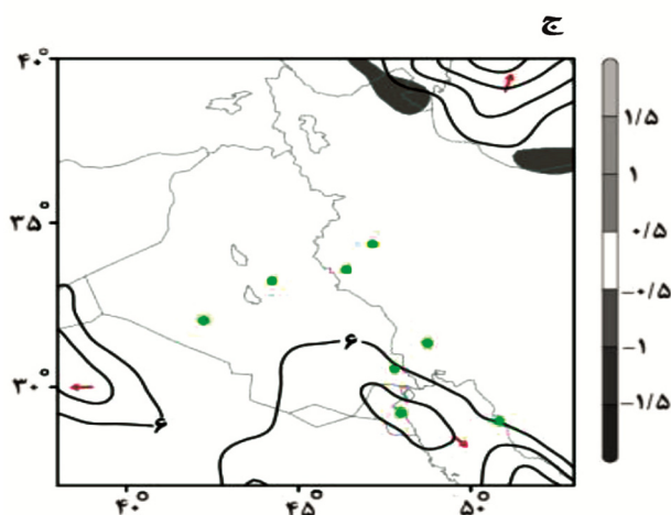
شکل ۶: گره‌های الف) فشار میانگین تراز دریا بر حسب hPa (خطوط توپر)، ارتفاع ژئوپتانسیلی تراز ۵۰۰ hPa بر حسب متر (خطوط به‌صورت خط چین) و پیکان‌های باد ده متری؛ ب) تصویر ماهواره MODIS؛ ج) سرعت باد بر حسب m/s (خطوط توپر) و مولفه قائم سرعت باد بر حسب pa/s (مناطق سایه زده) برای روز ۱۹ فوریه ۲۰۱۷
