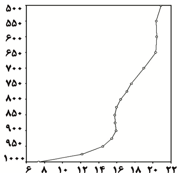
شکل ۹ ب: سطح مقطع قائم باد افقی و مولفه قائم باد (نواحی سایه زده شده) در عرض جغرافیایی ۳۲° شمالی و (ب) نیم‌رخ قائم مولفه قائم باد در عرض جغرافیایی ۳۲° و طول جغرافیایی ۴۳°، ساعت ۱۸ UTC روز ۱۷ فوریه ۲۰۱۷
