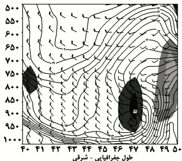
شکل ۹ الف: سطح مقطع قائم باد افقی و مولفه قائم باد (نواحی سایه زده شده) در عرض جغرافیایی ۳۲° شمالی و (ب) نیم‌رخ قائم مولفه قائم باد در عرض جغرافیایی ۳۲° و طول جغرافیایی ۴۳°، ساعت ۱۸ UTC روز ۱۷ فوریه ۲۰۱۷
