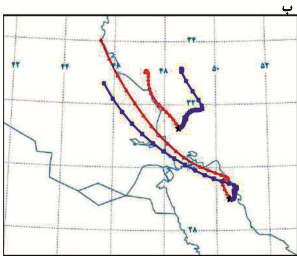
شکل ۸: برون‌دادهای الف) دید افقی مدل DREAM؛ ب) مسیر حرکت گرد و خاک مدل HYSPLIT (خط کم‌رنگ ارتفاع ۷۰۰ و خط پررنگ ارتفاع ۱۵۰۰ متری)، ۱۹ فوریه ۲۰۱۷
