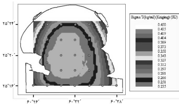
شکل ۸ - خطوط هم‌تراز انحراف معیار کریگیدن
