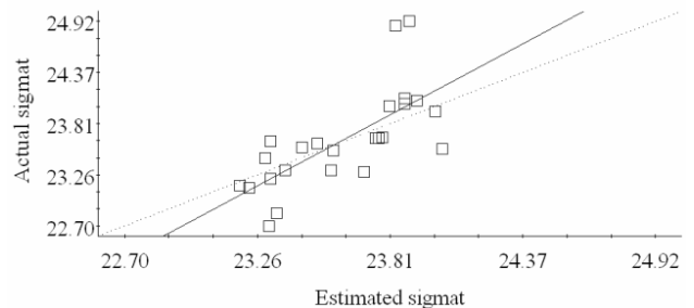
نمودار ۴- اعتبارسنجی متقابل به روش کریگیدن
