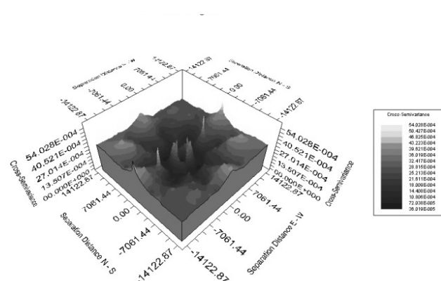
شکل ۳- روش سه بعدی تغییر نگار Sigma T
