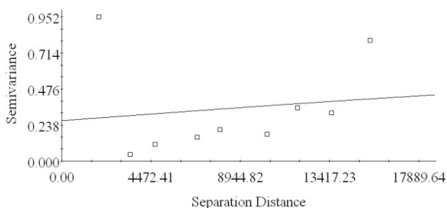
Isotropic Variogram (Sigma T)
