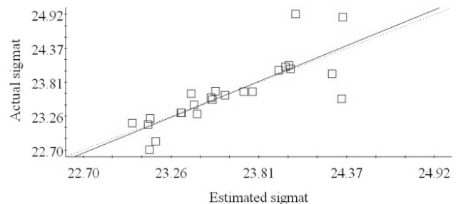
نمودار ۵- اعتبارسنجی متقابل به روش هم‌کریگیدن
