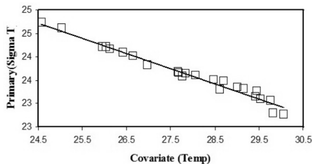
نمودار ۷- خط رگرسیون بین Sigma T و Temp
