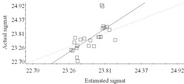
نمودار ۶- اعتبارسنجی متقابل به روش عکس فاصله‌ی موزون
