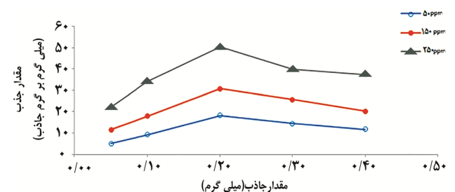
شکل ۲: تاثیر مقدار جذب بر جذب یون کادمیوم توسط جلبک گراسیلاریا
