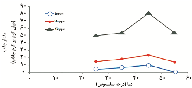
شکل ۳: اثر دما بر جذب یون فلزی کادمیوم توسط جلبک قرمز گراسیلاریا
